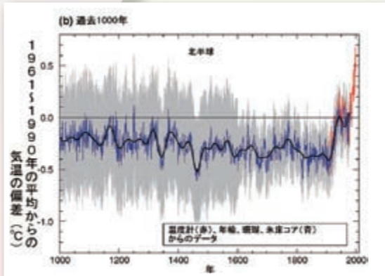
上図は、過去1000年の北半球の気温の変化です。過去100年で0.74℃気温が上昇しました。
